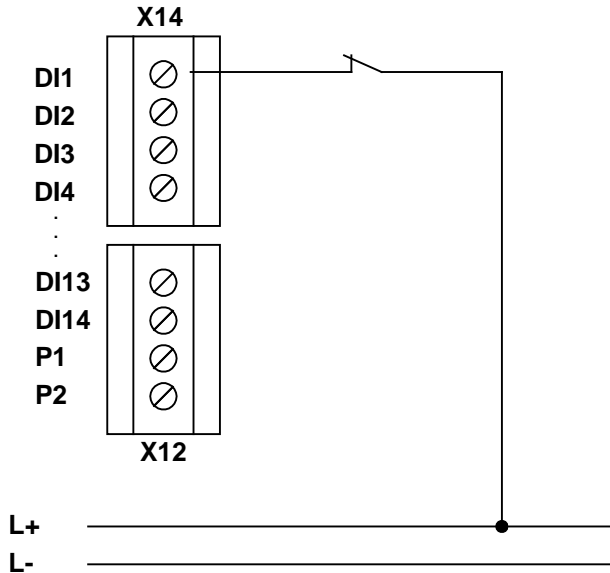
Bild: Einkanaliger Sensor, ohne Querschlussprüfung
