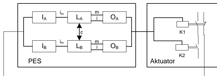
Einkanaliger Ausgang KSM mit intern zweikanaliger Verarbeitung(EAX) und zweikanaliger Aktuator mit mind. einkanaliger Diagnose
