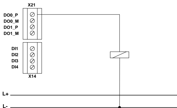
Bild: Einkanalig schaltender P-Ausgang.
