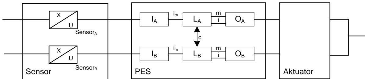
Zweikanaliges Sensorsystem mit getrennter Signalverarbeitung in zwei Kanäle, Diagnose durch Quervergleich in der PES
