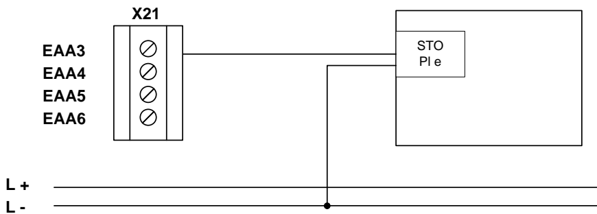
Bild: Zweikanaliger Ausgang in Verbindung mit Gerät mit geprüfter Abschaltung
