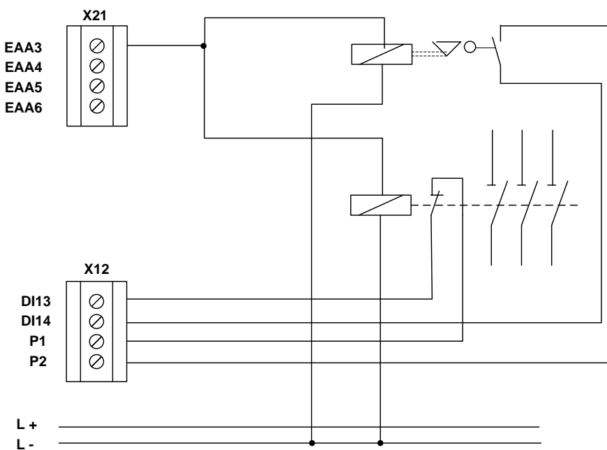
Bild: Zweikanaliger Ausgang in Verbindung mit zweikanaligem Abschaltkreis mit Testung
