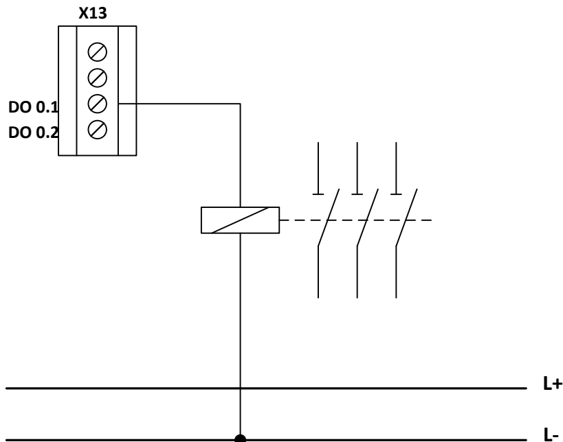
Bild: Beschaltung eines Hilfsausgangs
