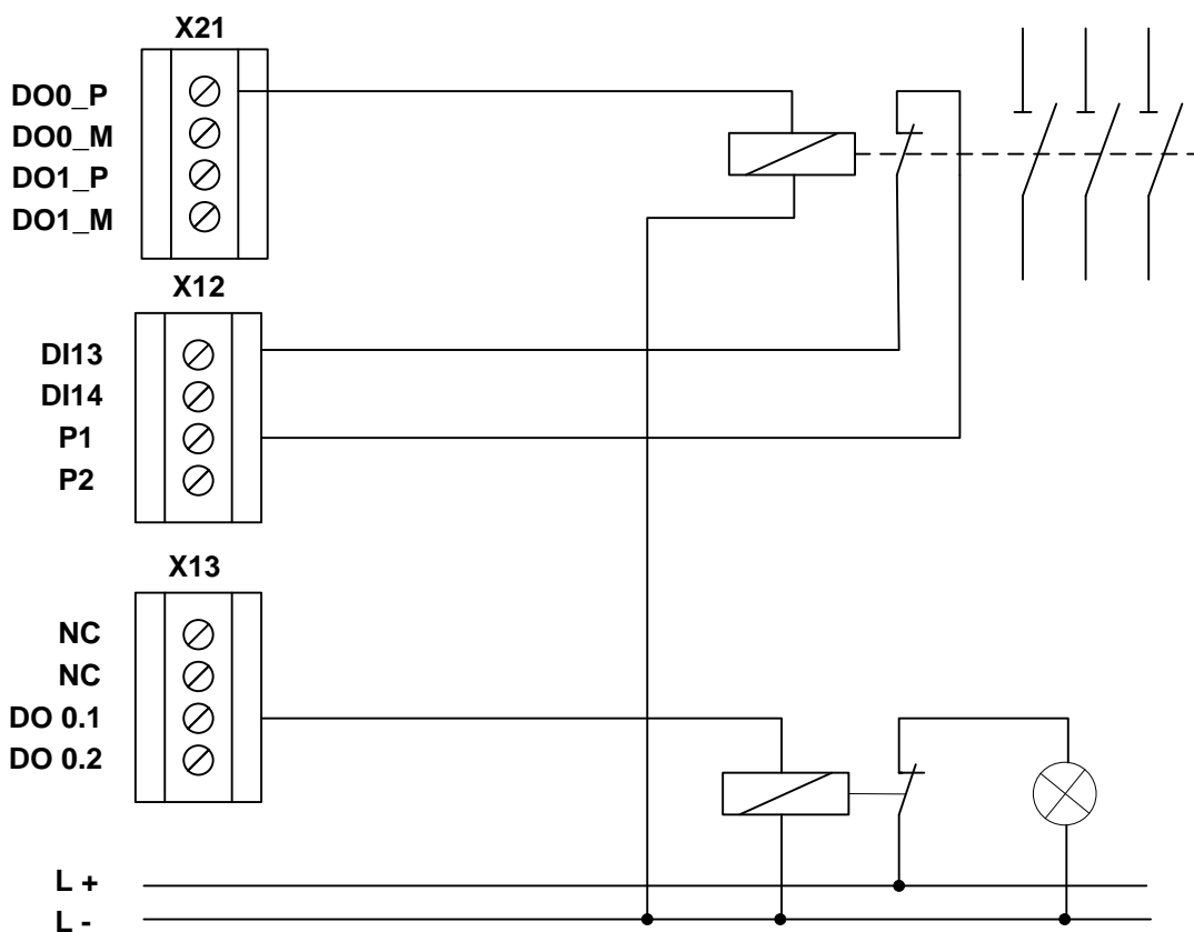
Bild: Einkanalig schaltender Relaisausgang mit Testung
