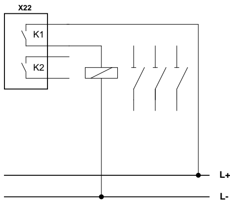
Bild: Einkanalig schaltender Relaisausgang.
