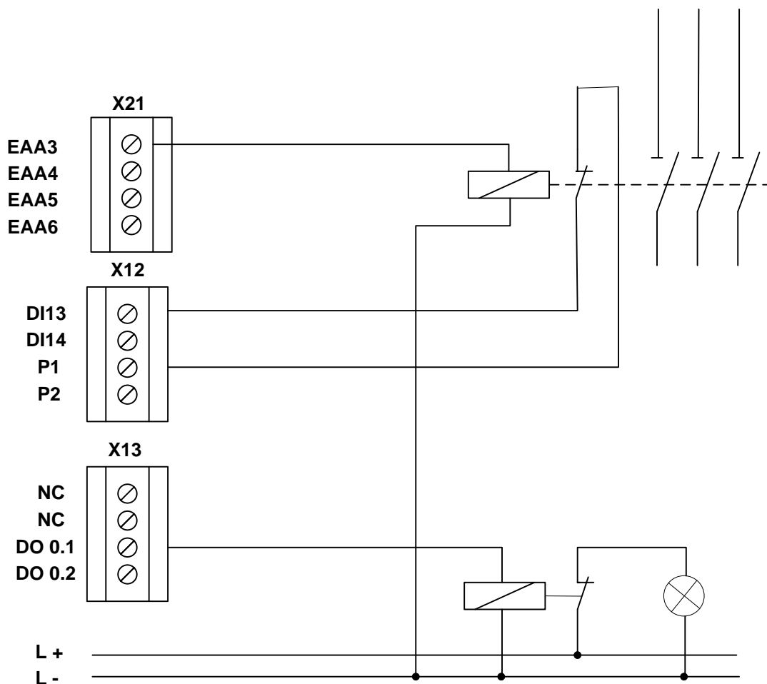
Bild: Zweikanaliger Ausgang mit einkanaliger Beschaltung mit Testung
