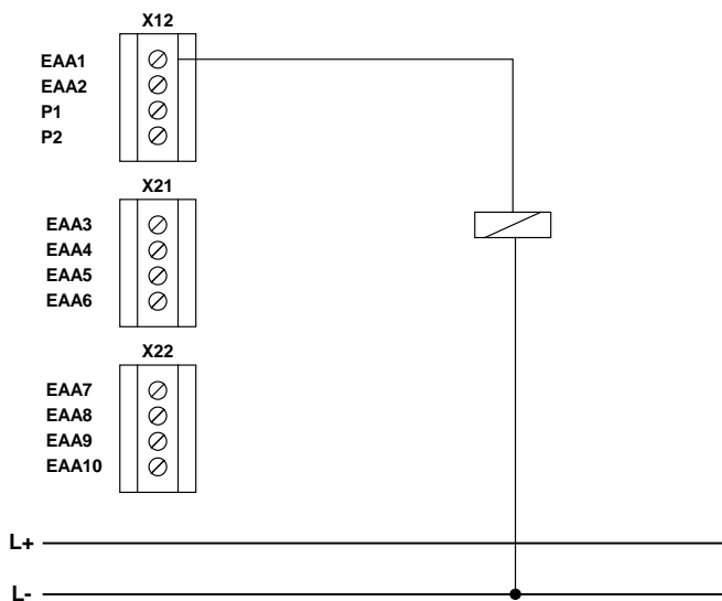
Bild: Zweikanaliger Ausgang mit einkanaliger Beschaltung ohne Testung
