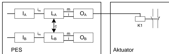
Einkanaliger Ausgang KSM und einkanaliger Aktuator ohne Diagnose
