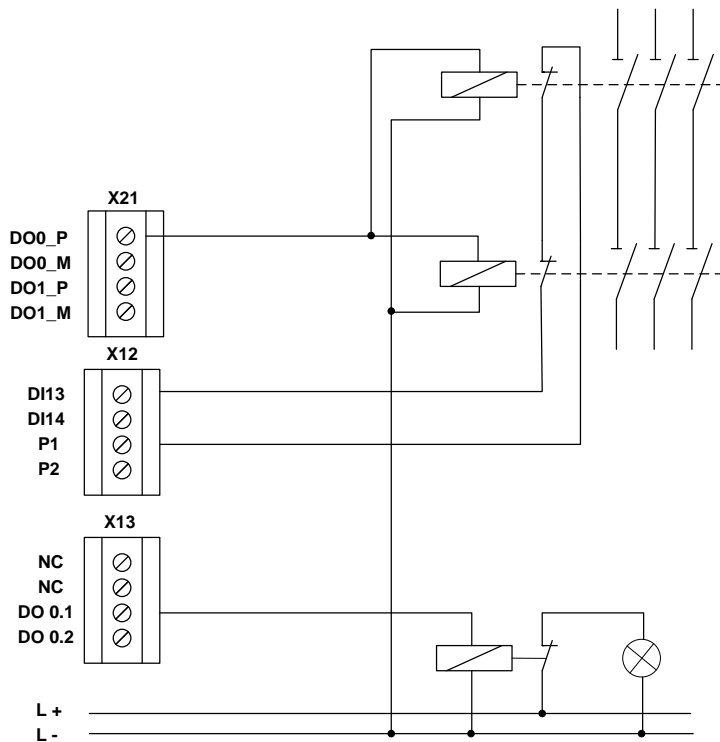
Bild: Einkanalig schaltender Ausgang DO 0_P mit zweikanaligem externem Kreis und Überwachung an Eingang 13 als Sammelrückmeldung
