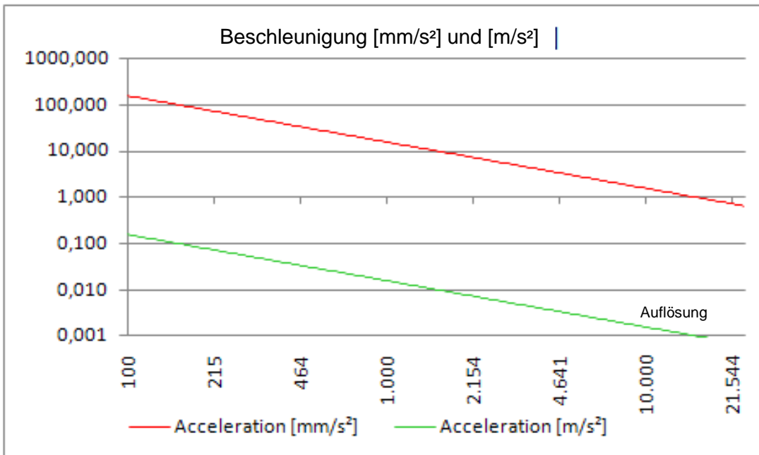
Grafik Beschleunigungsauflösung, linear (Werte in mm/s und m/s²)
