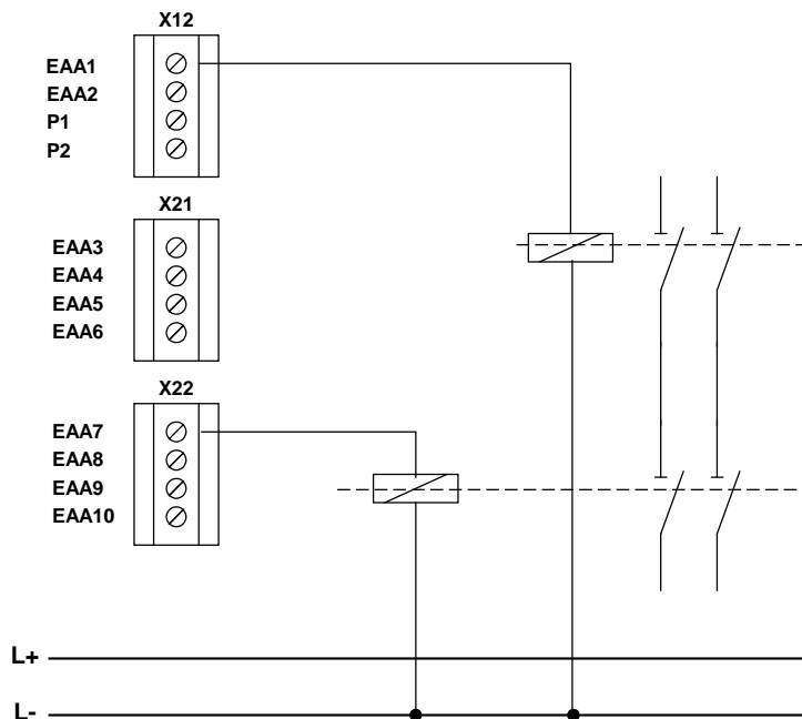
Bild: Redundante zweikanalige Ausgänge in unterschiedlichen Gruppen in Verbindung mit zweikanaligem Abschaltkreis
