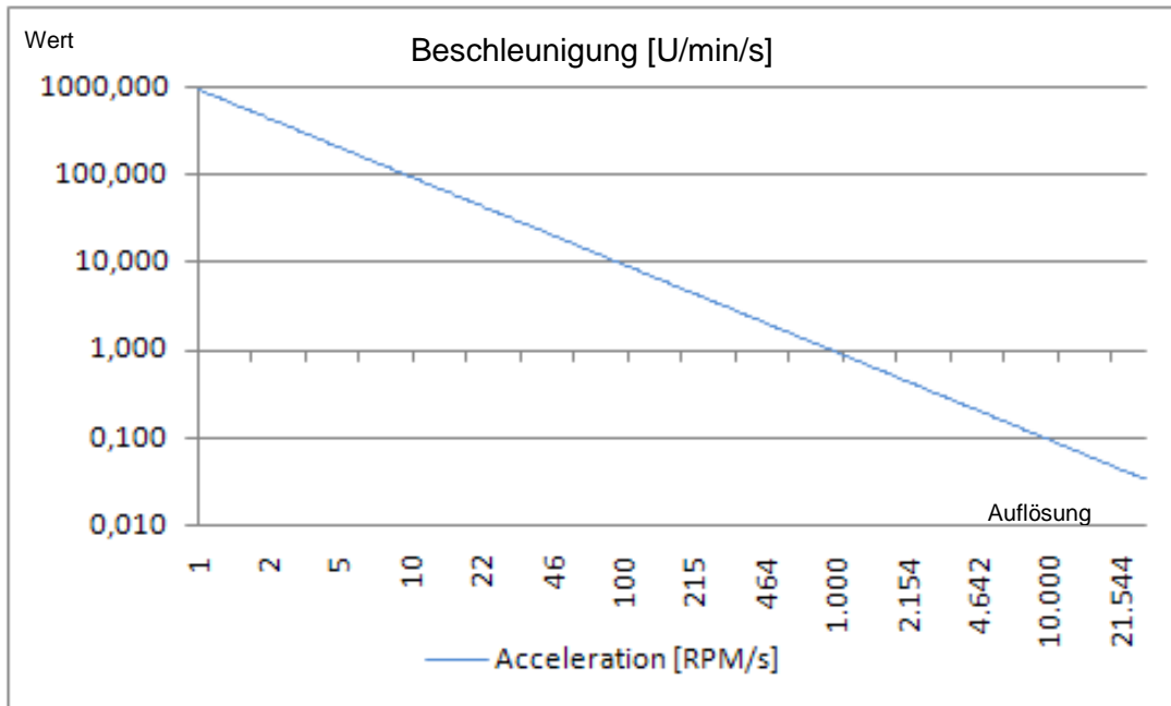
Grafik Beschleunigungsauflösung, rotatorisch (Werte in U/min/s)
