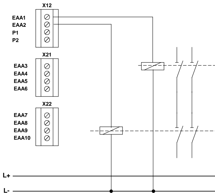
Bild: Redundante zweikanalige Ausgänge in gleicher Gruppe in Verbindung mit zweikanaligem Abschaltkreis
