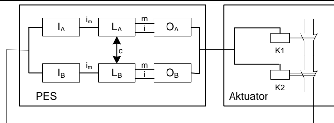
Einkanaliger Ausgang KSM mit intern zweikanaliger Verarbeitung (EAX) und zweikanaliger Aktuator mit zweikanaliger Diagnose
