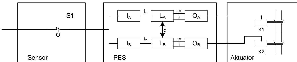
Einkanaliges Eingangselement und zweikanaliger Verarbeitung mit niedrigen bis mittleren DC durch Signalverarbeitung in zwei Kanälen und Diagnose mittels zyklischer Testung, PL / SIL abhängig von zulässigen Fehlerrückstellungen und Testrate des Eingangselements.
